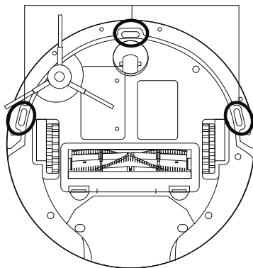
落下防止センサー
